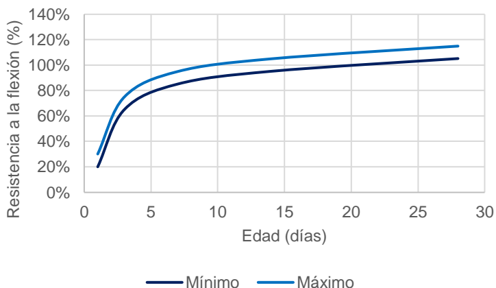
Desarrollo de resistencia en planta Alta Resistencia
